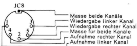
Draufsicht der DIN-Buchse
