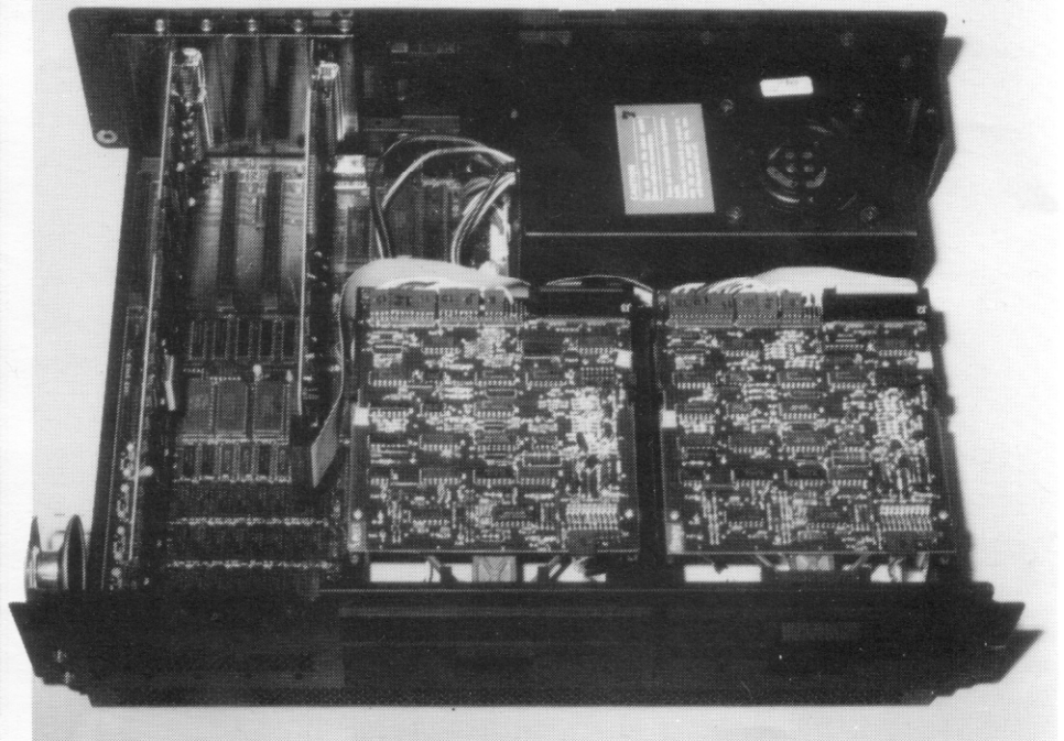
Afb. 2. In het interieur domineert de kolossale voeding. Links de vijf uitbreidingsconnectoren.
