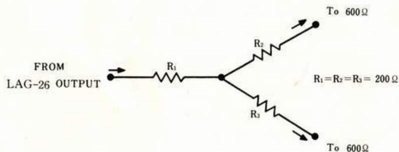
Fig. 2-2 Stereo input pad.
